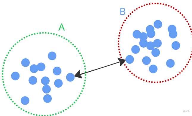
Figura 1.4 In questa figura è rappresentato il metodo di collegamento singolo in cui i punti colorati in blu sono i punti dati e la freccia rappresenta la distanza minima tra due punti di cluster diversi.
