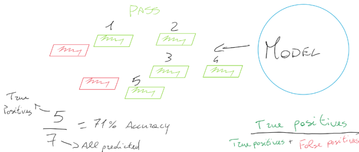
Figura 1.14 Nella figura è rappresentato uno schema per calcolare la precisione del modello.
