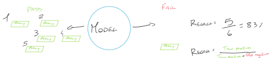
Figura 1.14 Nella figura è rappresentato uno schema per calcolare il recall del modello.
