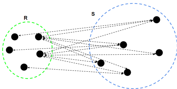
Figura 1.6 In questa figura è rappresentato il metodo di collegamento medio in cui i punti colorati in nero sono i punti dati e le frecce rappresenta la distanza tra le coppie di punti.
