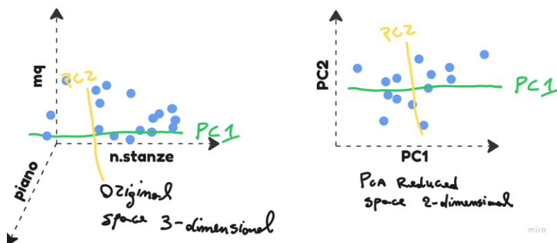
Figura 1.8 Riduzione delle feature grazie al PCA, lo schema a sinistra presenta 3 dimensioni numero di stanze, piano e mq, mentre quella a destra 2 dimensioni, ovvero PC1 e PC2 che PCA ha calcolato.
